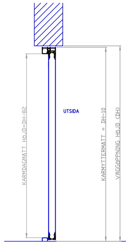
VERTIKALSEKTION
