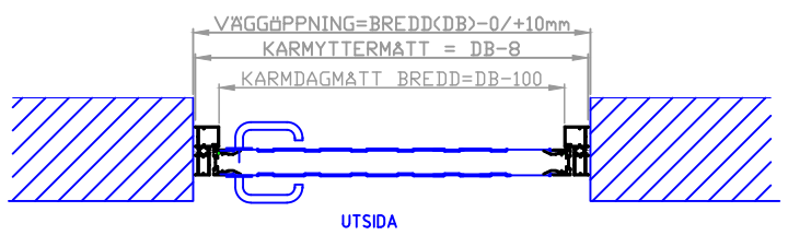
A-A HORIZONTALSEKTION
